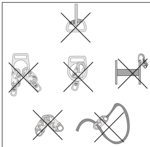
FIGURA 4 - CONEXIONES INCORRECTAS
